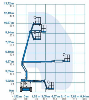
Diagrama de trabajo Z-34/22 IC
